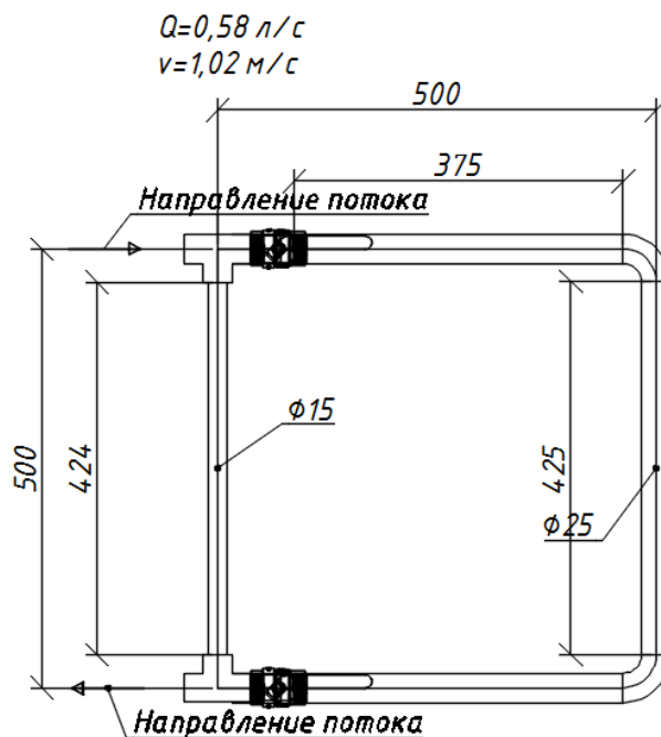
Рисунок 1 – Схема полотенцесушителя
