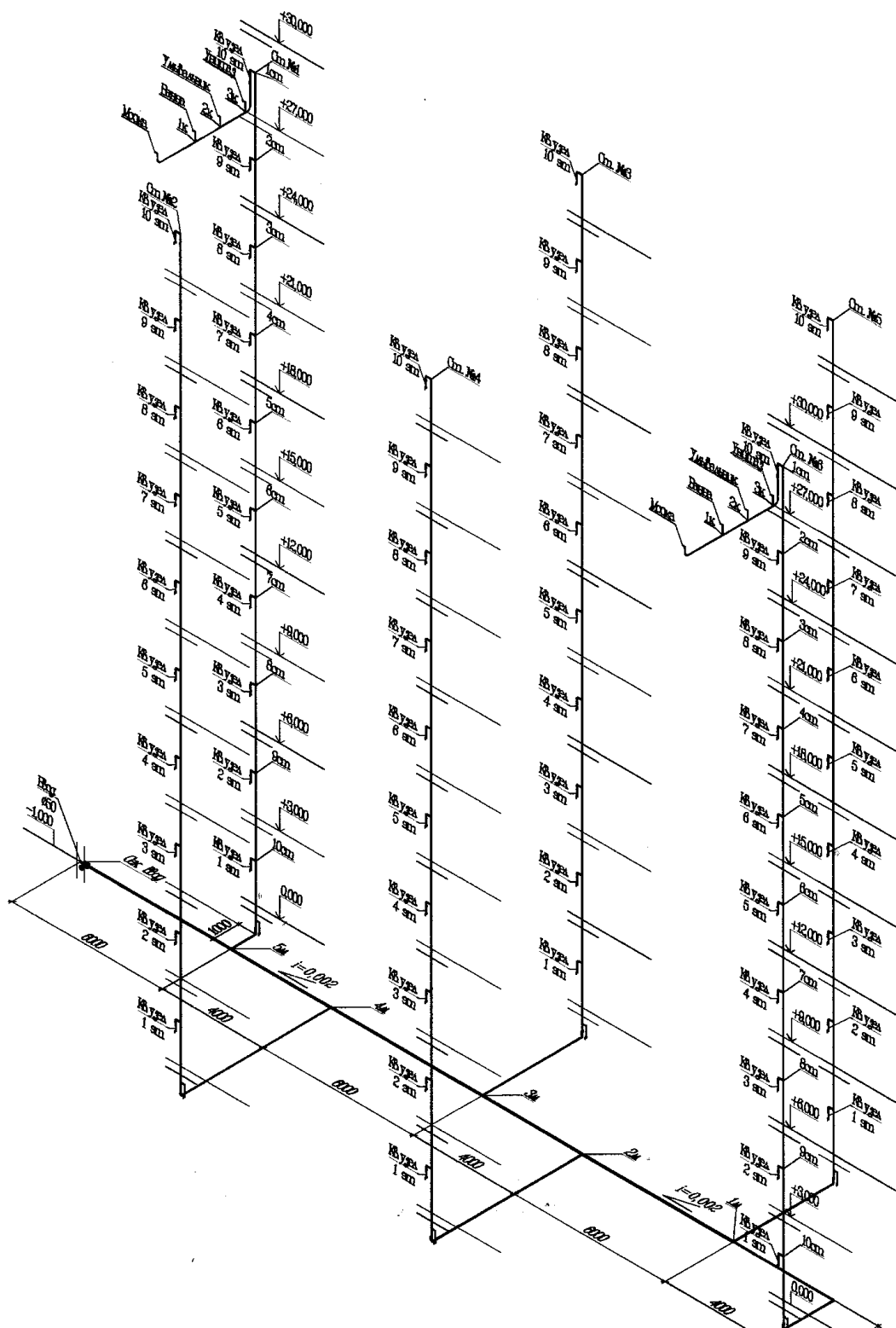
Рисунок 2 – Схема системы холодного водопровода
